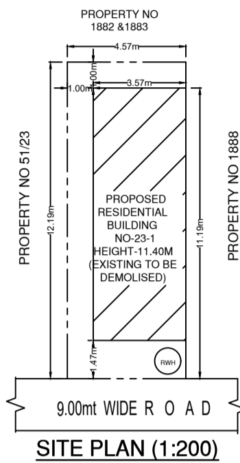
SITE PLAN (1:200)
