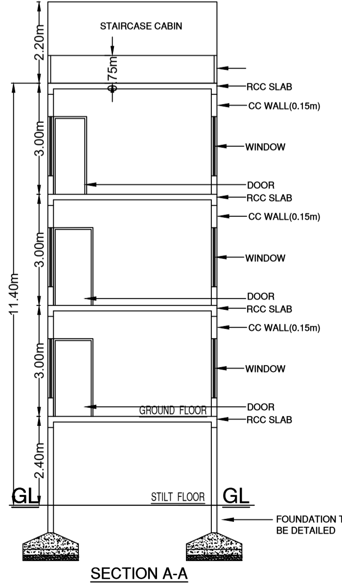
SECTION A-A
